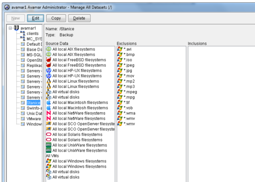
Obrázek 22: Datasets detail
