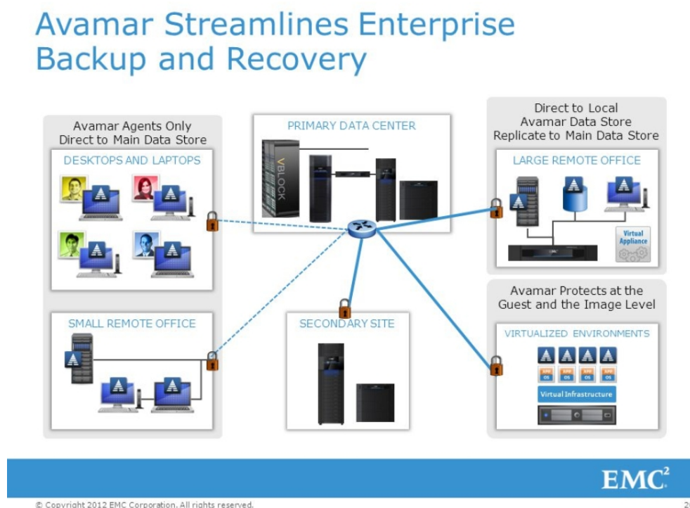
Obrázek 9: EMC Avamar [9]
