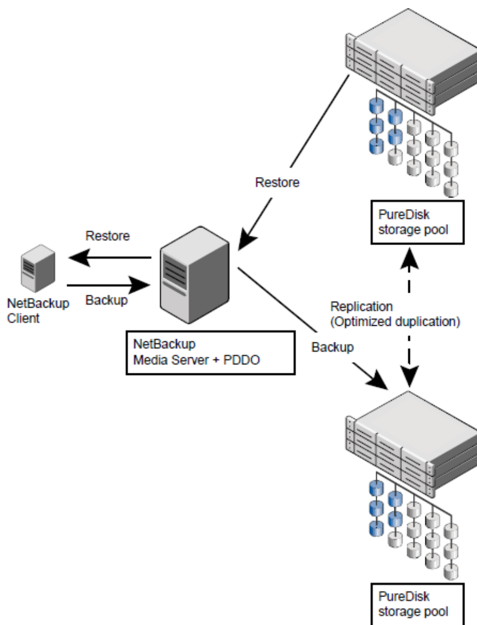
Obrázek 16: Replikace dat [15]
