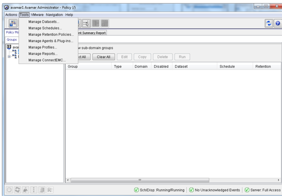
Obrázek 21: Datasets
