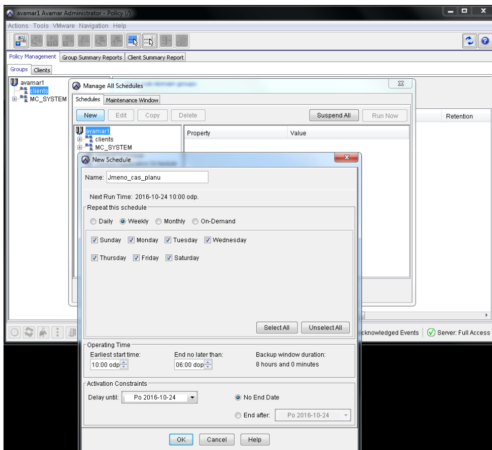
Obrázek 23: Schedules
