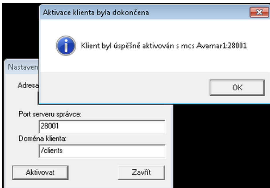
Obrázek 26: Úspěšná aktivace
